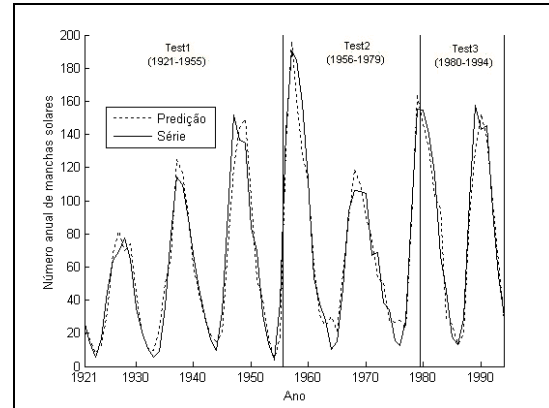
Figura 5.3 – Preditor treinado pelo PPL sem seleção de entrada
