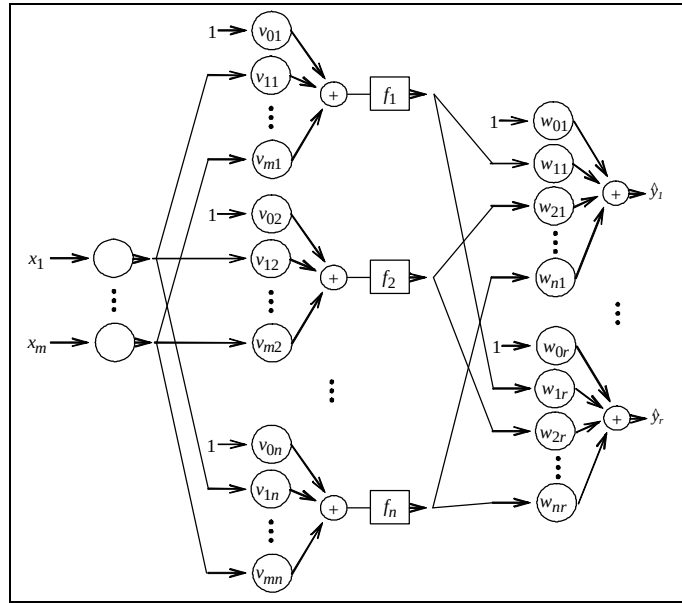
Fig. 2.1 – Rede neural artificial tipo feedforward com uma camada intermediária
