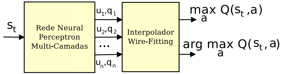
Fig. 4.5: Arquitetura “Wire-Fitting-Neural- Q ” no cálculo da ação máxima
