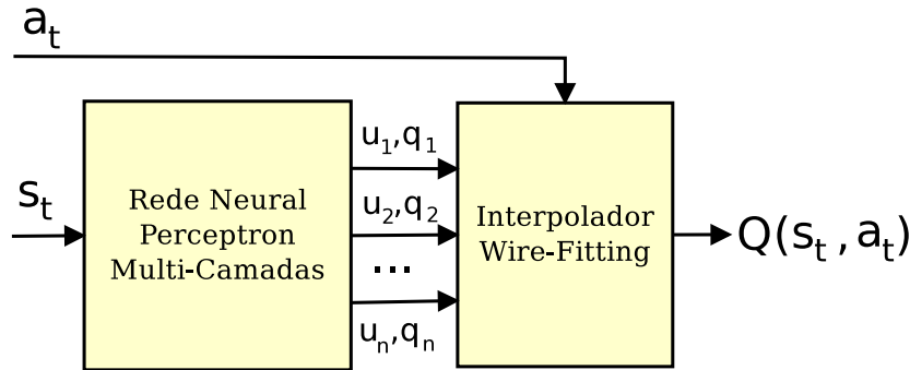
Fig. 4.4: Arquitetura “Wire-Fitting-Neural-Q”
