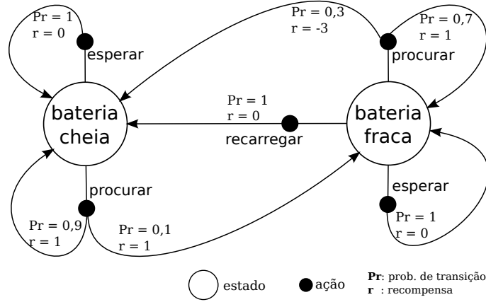
Fig. 2.1: Exemplo de um sistema de Markov de um robô lixeiro. Definem-se dois estados: “bateria cheia” e “bateria fraca”; e três ações: “esperar”, “procurar” e “recarregar”.
