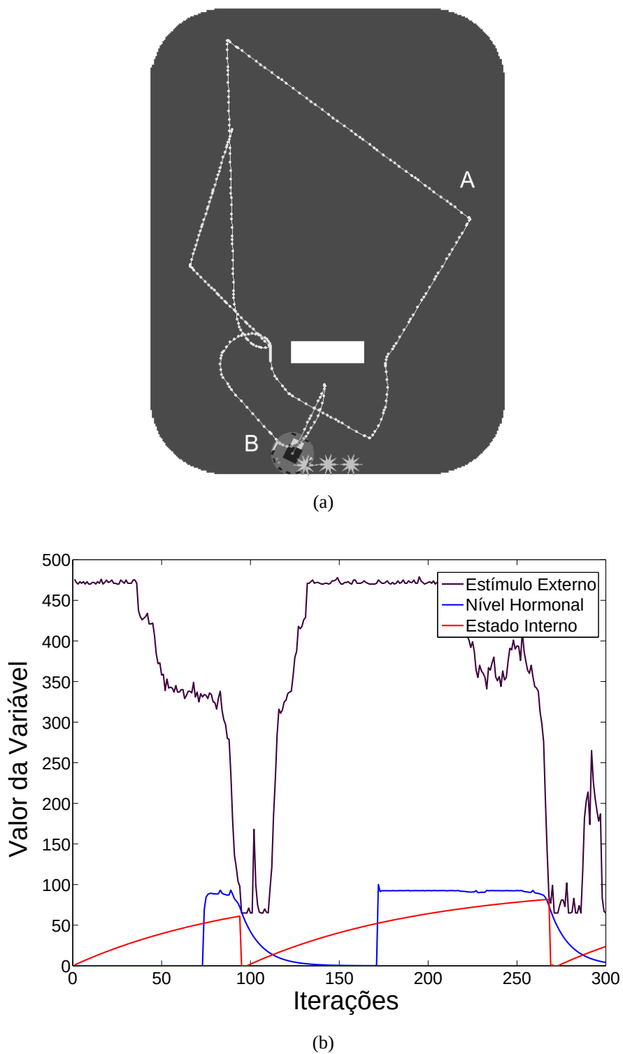
Fig. 4.16: Trajetória (a) e dinâmica das variáveis (b) para SHAE-R. O ponto A indica o momento em que o hormônio começa a ser produzido pela segunda vez, e o ponto B indica o momento em que o robô aproxima-se da fonte luminosa, simbolizando a recarga de suas baterias.
