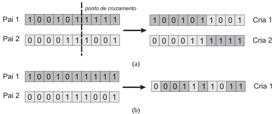
Fig. 2.4: Crossover de um ponto (a) e crossover uniforme (b) (reproduzido de Barra (2007), com permissão do autor)
