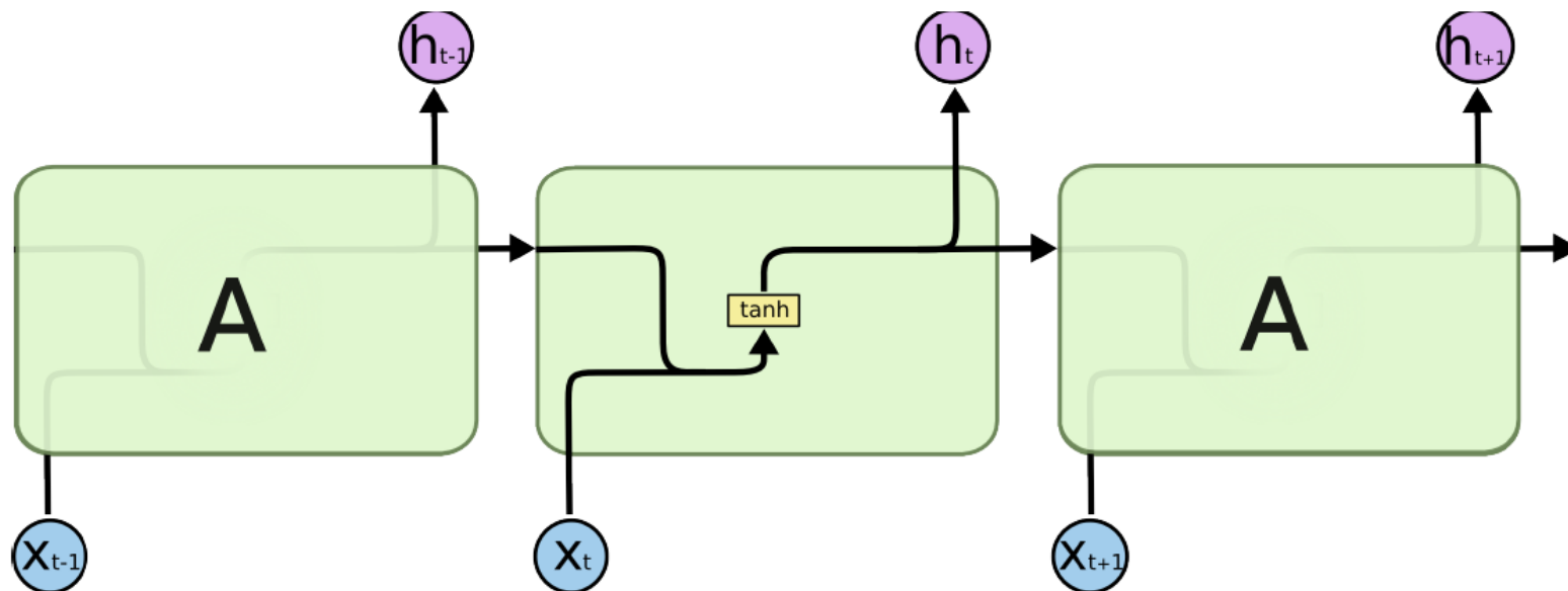
Figura 6 – Bloco de uma rede neural recorrente convencional com realimentação externa.
