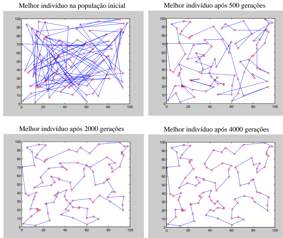
Figura. Solução de um problema de caixeiro viajante.
