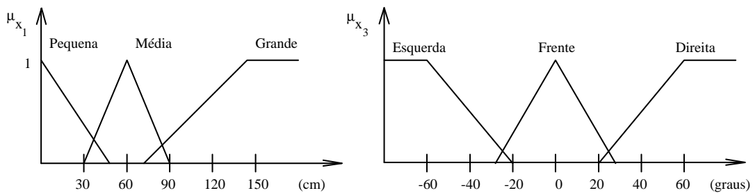
Figura 18 - Funções de Pertinência para variáveis x_1 e x_3
