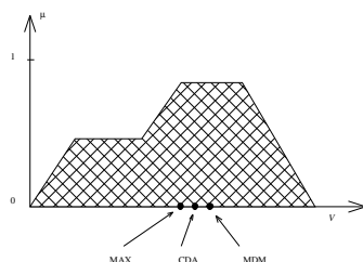
Figura 11 - Métodos de Defuzzyficação
