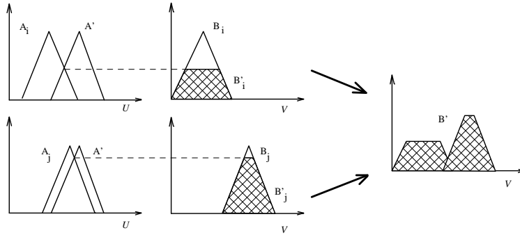
Figura 4: Mecanismo de Inferência Fuzzy
