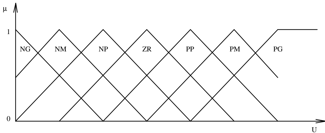
Figura 21 - Funções de Pertinência
