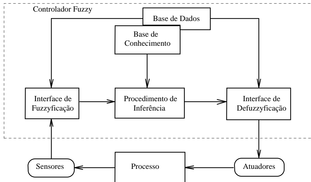
Figura 10 : Estrutura Básica de um Controlador Fuzzy
