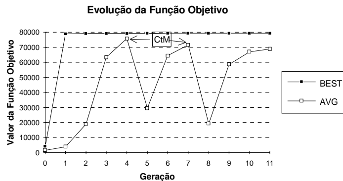
Figura 25 - Evolução da Função Objetivo
