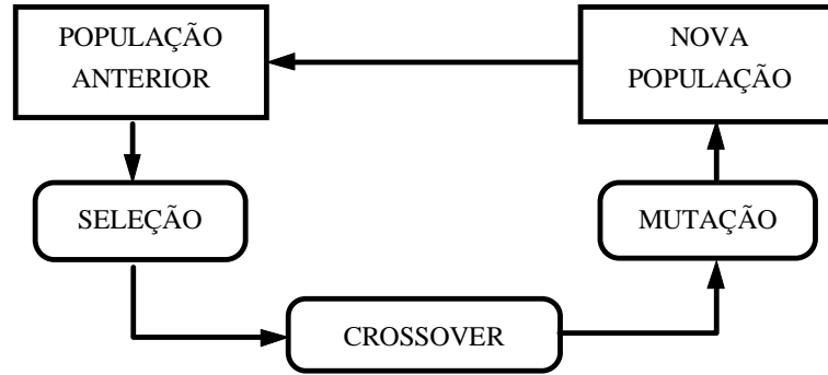
Figura 23 - Ciclo Básico de Algoritmo Genético
