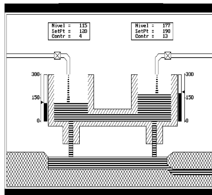
Figura 20 - Sistema de 2 Tanques Acoplados
