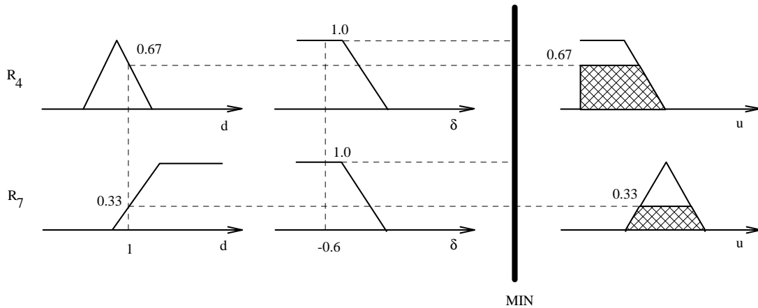
Figura 15 - Inferência : Composição MAX-MIN
