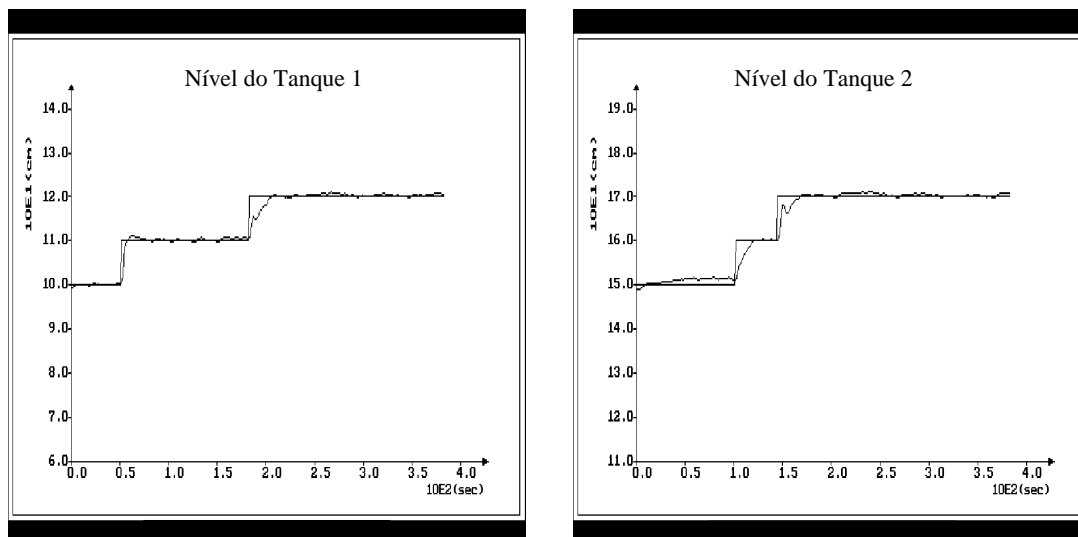
Figura 22 - Resultados para os Tanques
