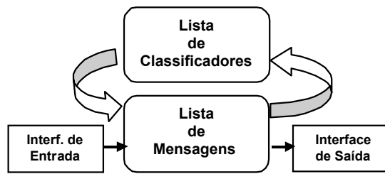
Figura 2.1: Sistema Classificador, Nível Básico
