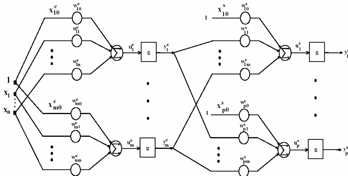
Figura 3.2: Perceptron de três camadas (uma camada intermediária)
