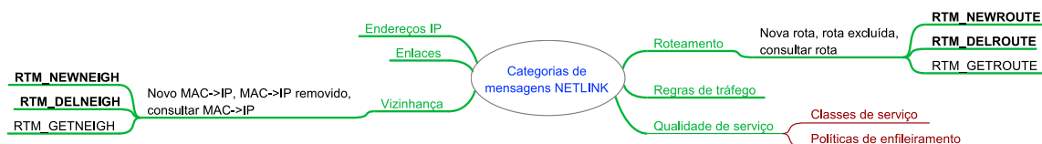
Figura 17: Hierarquia de mensagens RTNETLINK, com destaque para aquelas tratadas pelo daemon RF-Slave.
